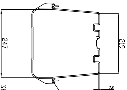
SEZIONE A-A
